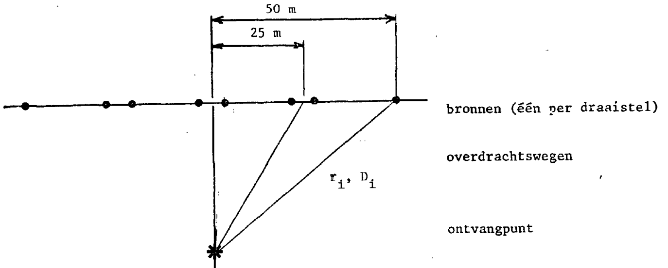
Figuur 1 : De gekozen bronplaatsen (materieel 64) en de bijbehorende overdrachtswegen
