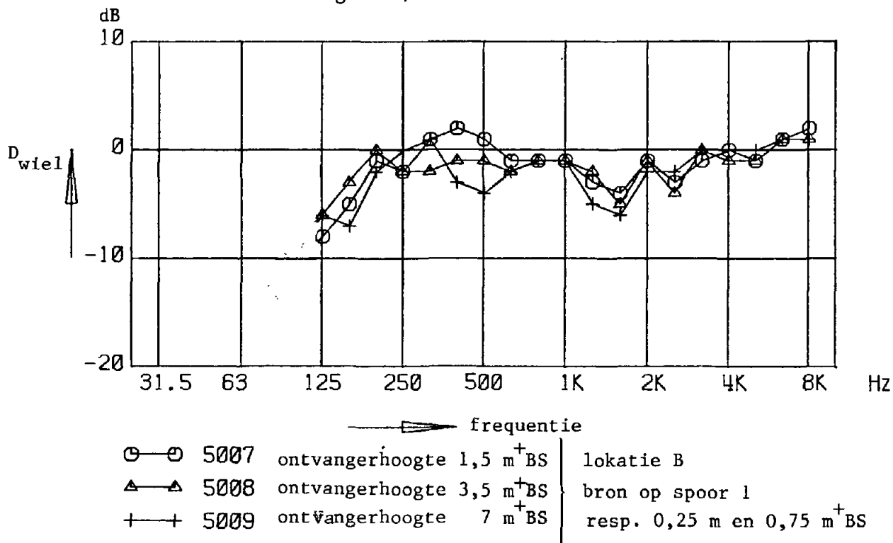
Figuur 8: De gemiddelde overdrachtsverzwakking voor een remmend wiel op spoor 1 uitgaande van twee evensterke puntbronnen op respectievelijk 0,25 en 0,75 m + BS naar verschillende waarneemhoogten op 15 m afstand van spoor 1.
