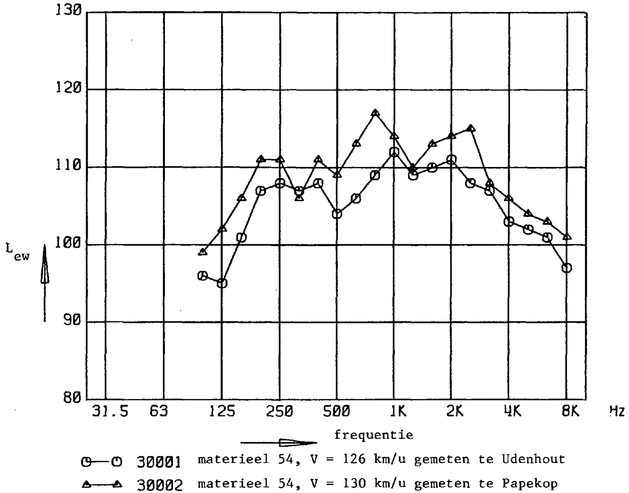
Figuur 12: Equivalente geluidvermogniveaus per draaistel bepaald uit metingen van het maximale geluiddrukkniveau op 25 m afstand van spoor 1 bij vier-wagenstellen van materieel 54.
