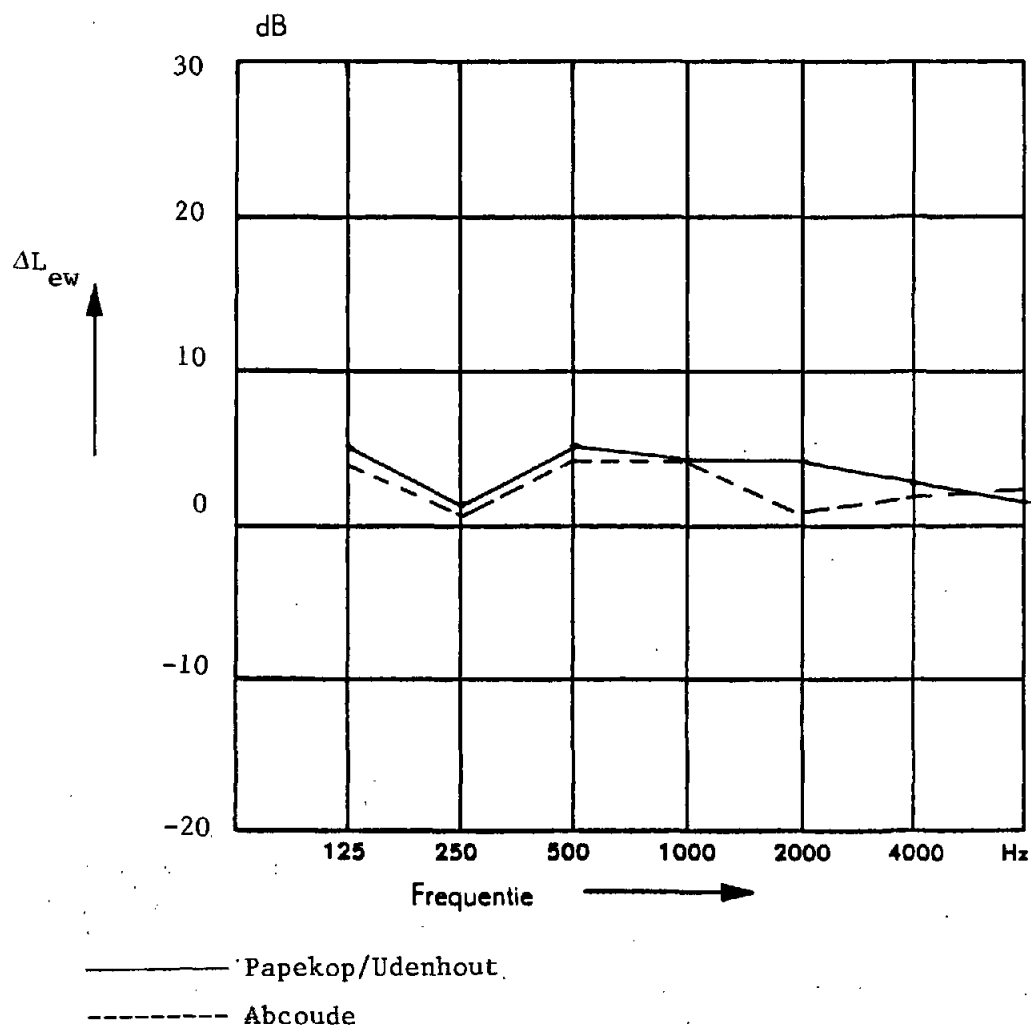
Figuur 13: Niveaunderschil in oktaafbanden van het geluidvermogeniveau per draaistel van een trein rijdend op een baan met houten dwarsliggers en rijdend op een baan met betonnen dwarsliggers.
