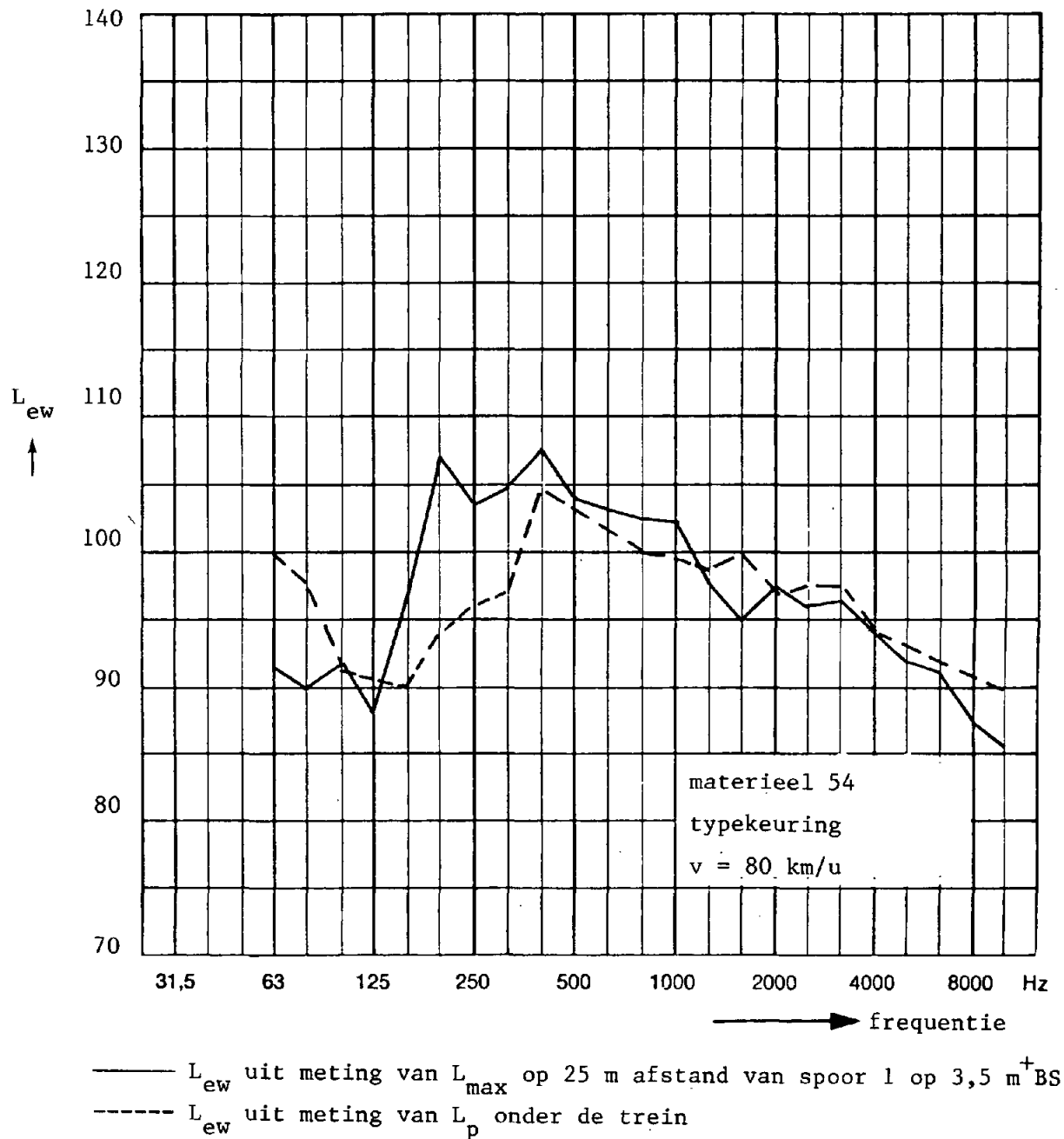
Figuur 21: Equivalente geluidvermogeniveaus per draaistel van materieel 54 volgens typekeuring bij 80 km/u. Vergelijking van bronniveaus bepaald uit metingen langs de baan en uit metingen onder de trein.
