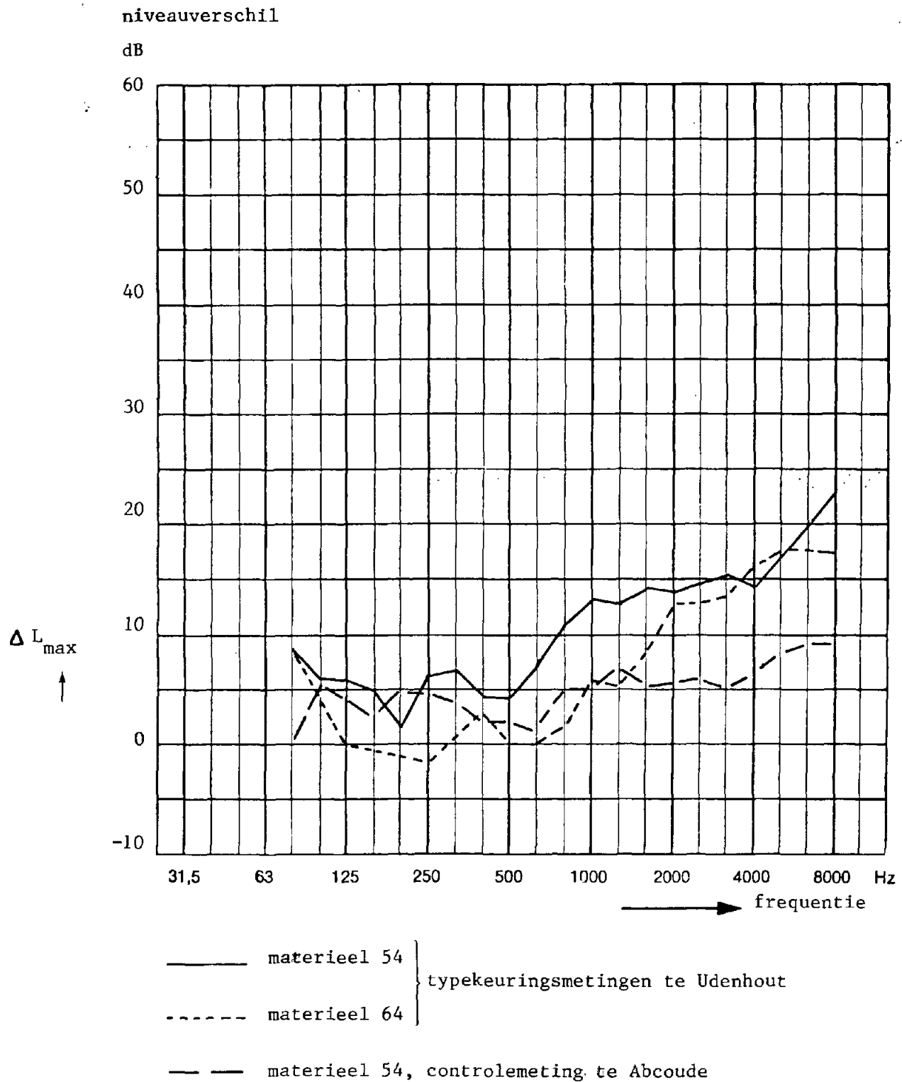
Figuur 17 : Niveautoename in de geluidemissie t.g.v. het remmen bij zowel typekeuringen- als dienstregelingsreinen. De verschillen zijn bepaald uit metingen van het maximale geluiddrukkniveau op 25 m afstand van spoor 1 (3,5 m + BS) tijdens de passage van treinen. De verschillen hebben betrekking op bedrijfsremmingen met een vertraging van ca. 0,5 m/s 2 .
