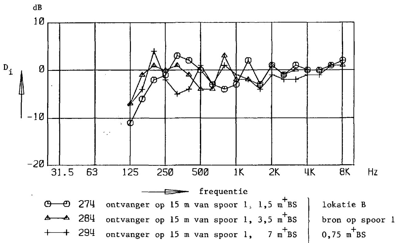
Figuur 7: De overdrachtsverzwakkingen van één puntbron boven spoor 1 naar verschillende waarneemhoogten op 15 m afstand van spoor 1.
