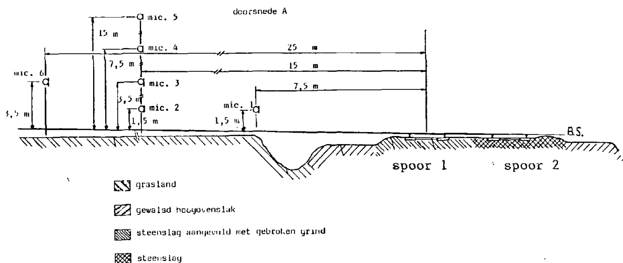
Figuur 3a : Dwarsdoorsnede en microfoonposities tijdens remmetingen bij lokatie A (komt overeen met lokatie B).
