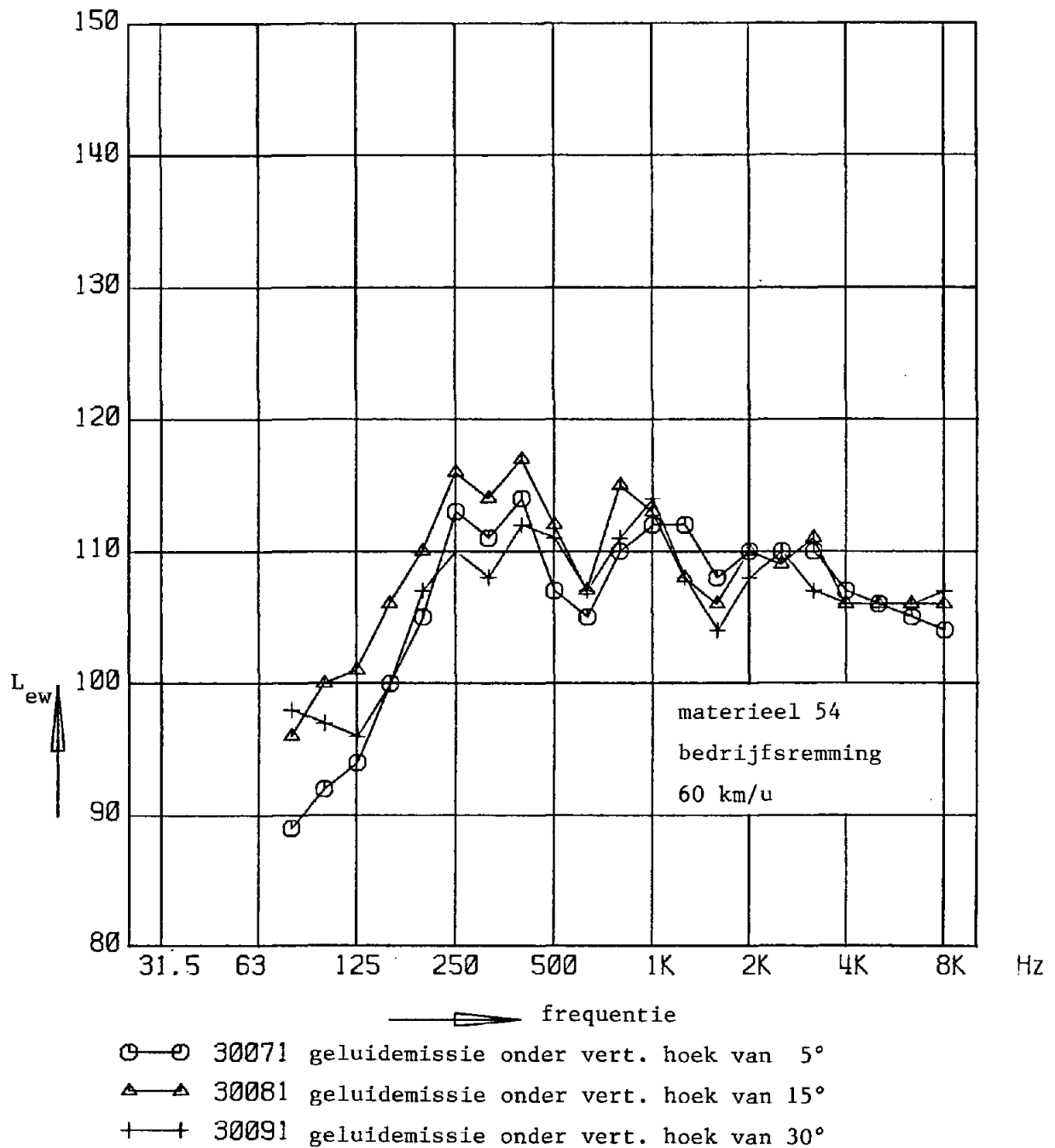
Figuur 15 : Immissierelevante bronsterkte per draaistel bij bedrijfsremming bepaald uit maximale geluidrukniveaus op 15 m afstand van spoor 1 op respectievelijk 1,5 m, 3,5 m en 7 m + BS.
