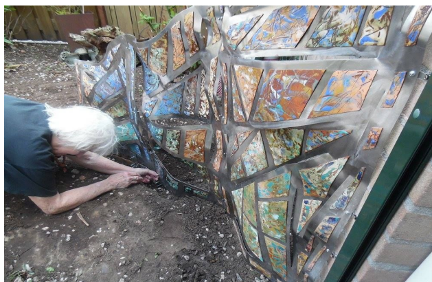
Montage van de waterslag op ingegraven fundament.
