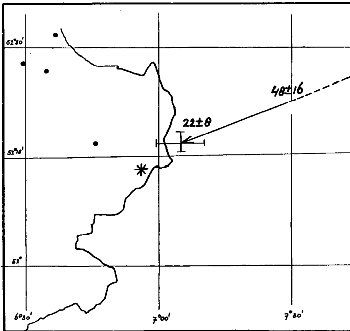
Figure 3: Grondtraject met hoogteaanwijzingen van het met FIRBAL berekende traject. Het hele lichtspoor heeft zich boven Duits grondgebied bevonden. Het inslagpunt te Glanerbrug is met een sterretje aangegeven.
