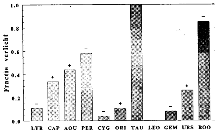
Figure 2: Maanfase tijdens de zwermmaxima in 1990
